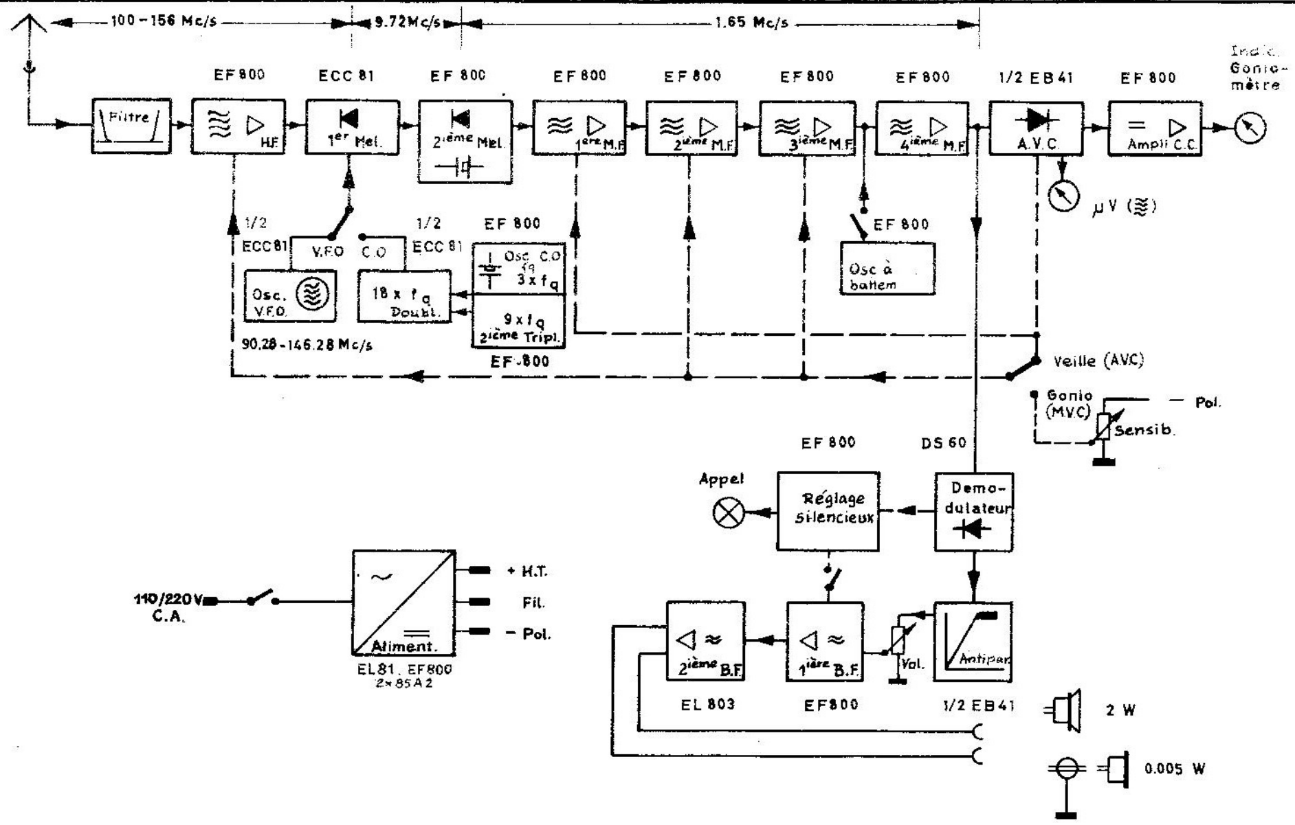
Récepteur V.H.F. NE 2
